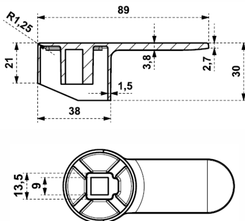
Tozzo 30mm | Tozzo 30mm
