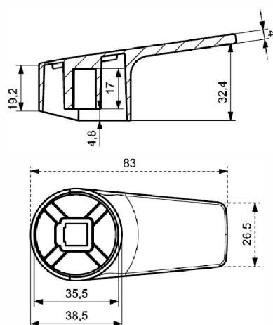
Single Lever - Mini Punch 30mm
